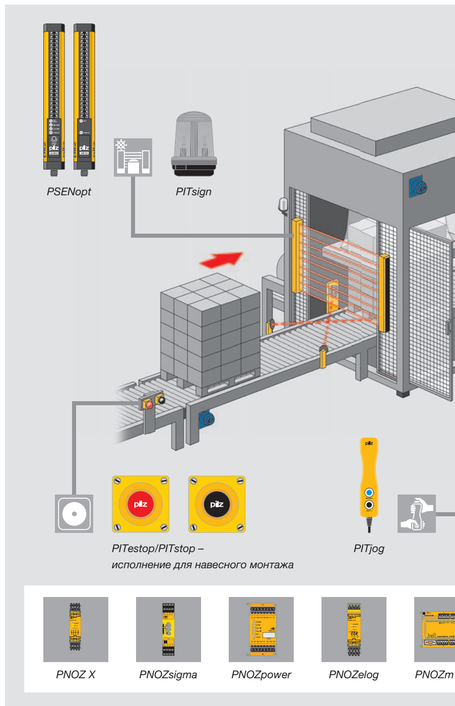
Типовой пример применения управляющих и сигнальных PИT - устройств от PILZ
